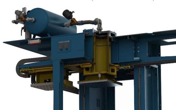
unidade de sopro e gasagem móvel unidade de sopro com tela de sopro
